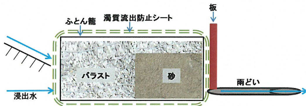
図 3-3 ふとん籠断面図 (横)
