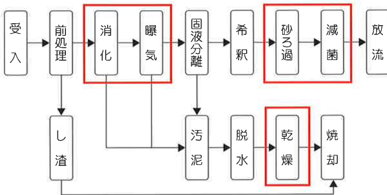
ぎ の わんせいすいえん しやうり 【宜野湾清水苑の処理フロー】
